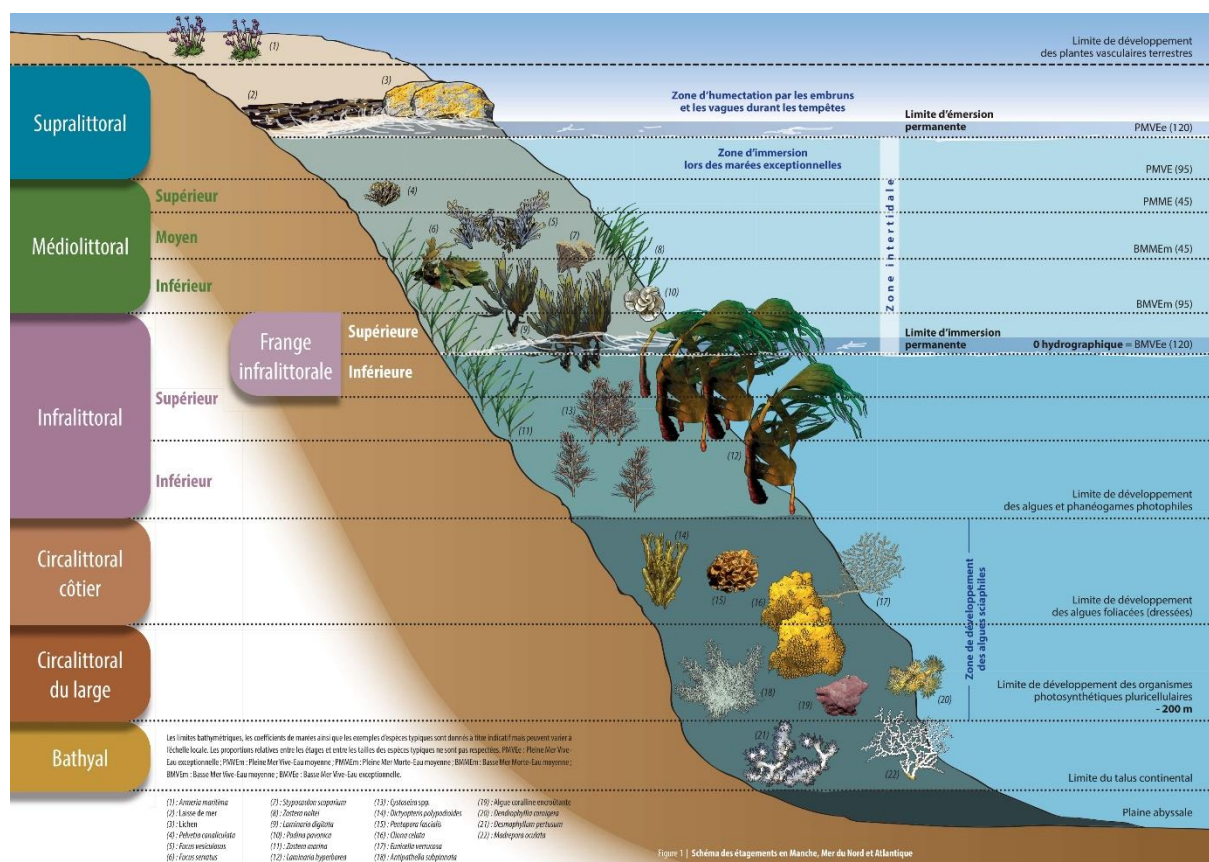
Figure 17 : Étagement en milieu marin
