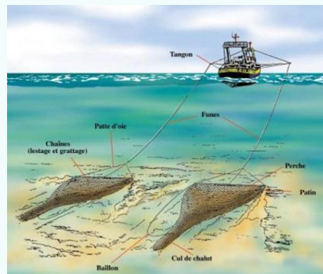
Figure 10 : Chalut à perches (Source : Ifremer).
