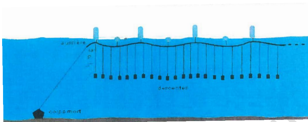
Figure 57 : Extrémité de filière subflottante (Source : avis d'enquête publique « lotissement de cultures marines » sur l'extension de la zone de concessions pour élevage de moules sur filières au large de Leffrinckoucke-Zuydcoote)
