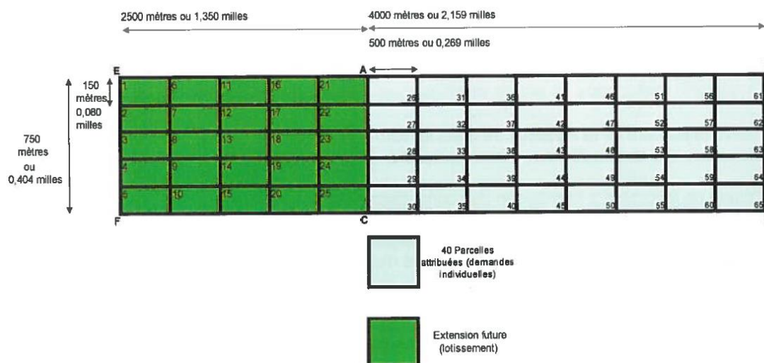
Figure 56 : Zone de captage et élevage de moules sur filières – plan des installations (mars 2006) (Source : DDTM 59)
