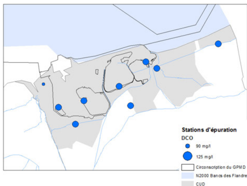
Demande Chimique en Oxygène (DCO)
