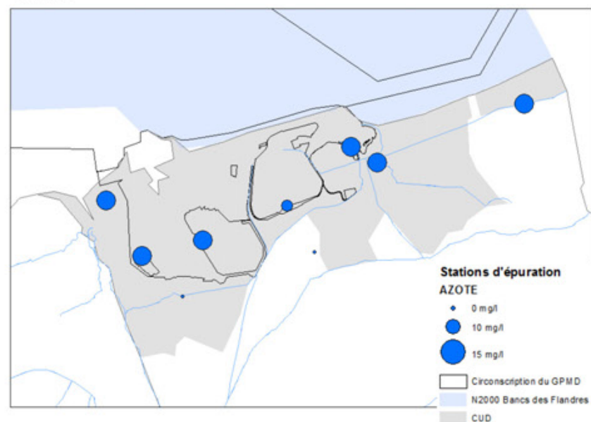
Azote
