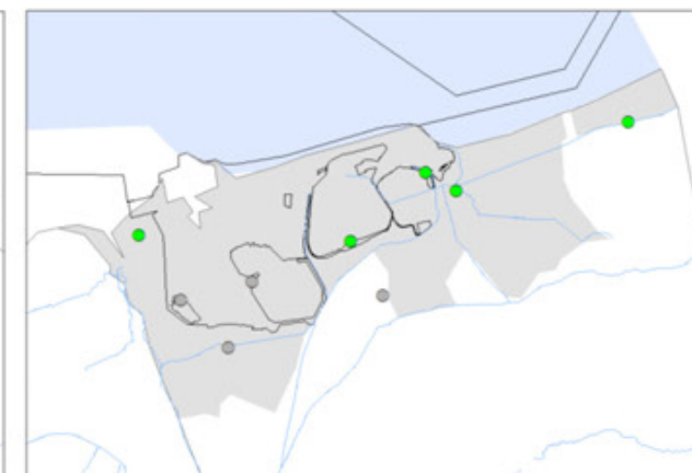
Métaux
