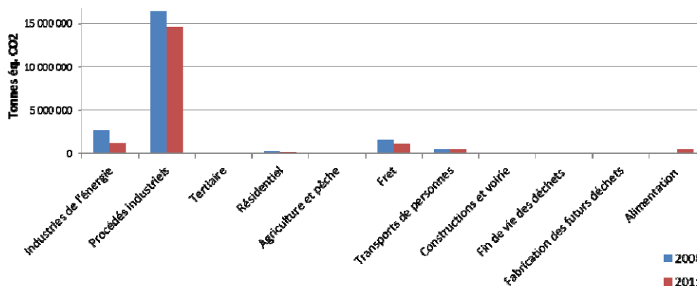
Evolution de bilan carbone « territoire » de la Communauté urbaine de Dunkerque entre 2008 et 2011 du Plan Climat Energie Territorial (CUD, 2014)
