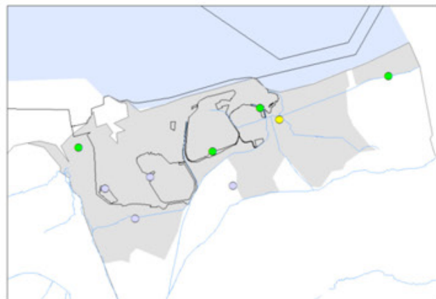
Pesticides urées carbamates
