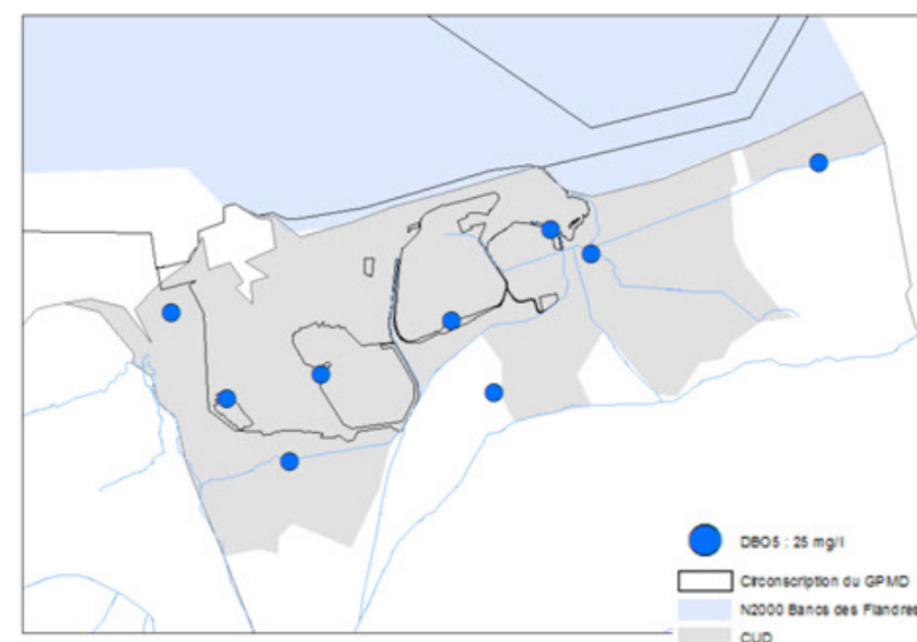
Demande Biologique en oxygène sur 5 jours (DBO5)
