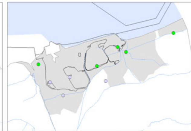
Composés organiques volatils
