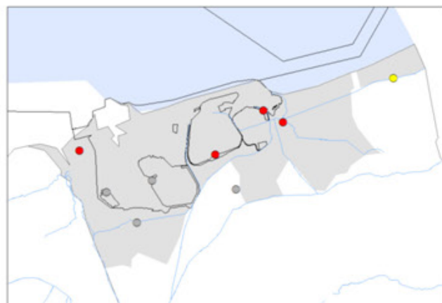
Composés phénoliques
