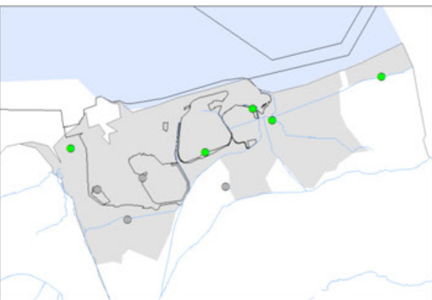
Composés benzéniques
