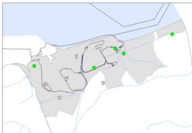
Herbicides divers
