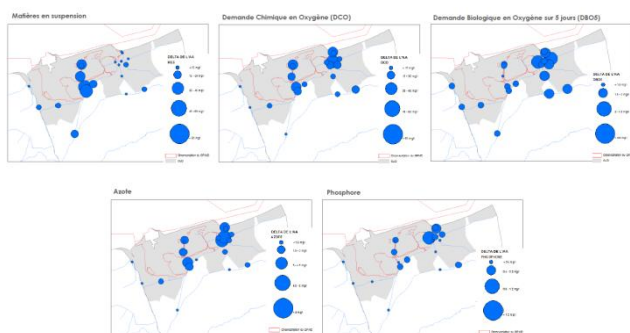
Planche : Analyses des eaux superficielles sur les paramètres NQE pour la zone du delta de l'Aa à proximité du site Natura 2000 des Bords des Flandres
