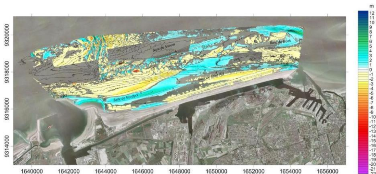
Différentiel bathymétrique de l'avant-côte de l'UG4 entre 2000 et 2013 (Hequette et al., 2014)
