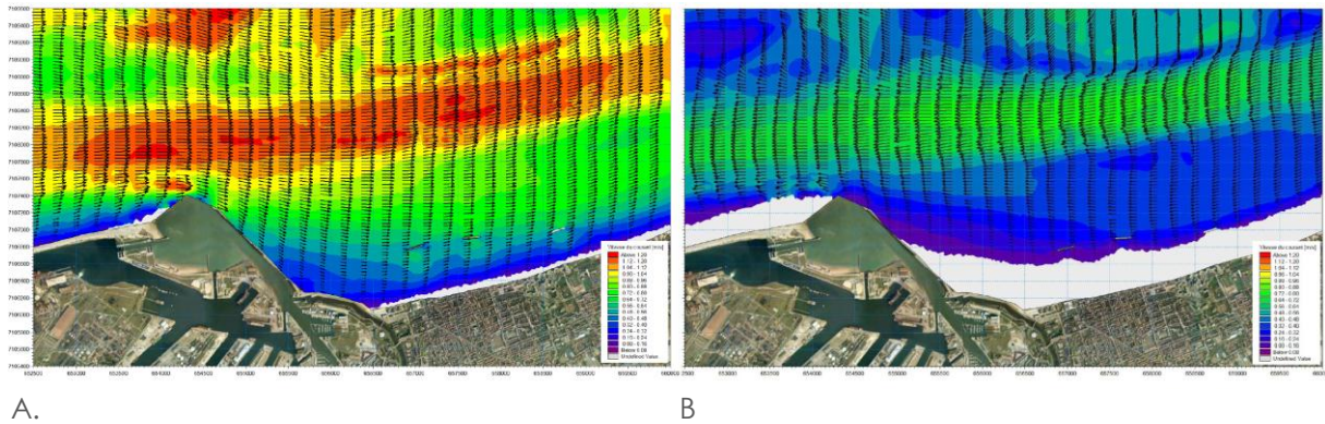
Direction et force des courants de marée à marée montante (A) et à marée descendante (B) de vive-eau (DHI, 2012)
