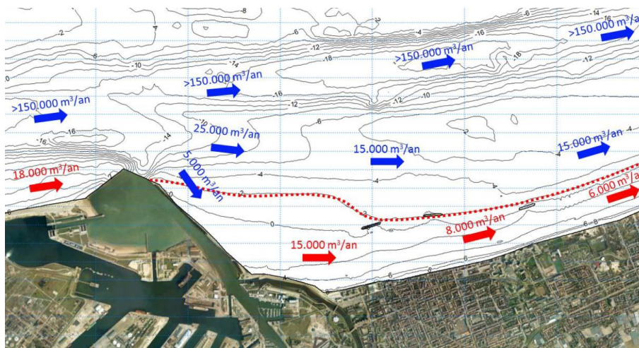
Transport sédimentaire sur le secteur de la Digue des Alliés, induit par les courants de houle (rouge) et courants de marée (bleu). La limite d'action des houles (isobathe -2m CM) est indiquée par le trait en pointillé rouge (DHI, 2012)
