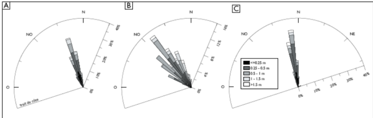
Roses des houles enregistrées sur l'estran à Malo-les-bains de part et d'autre du brise-lame Est en novembre 2004 (A : Ouest du brise-lame, B : arrière, C : Est) (Oblinger, 2008)
