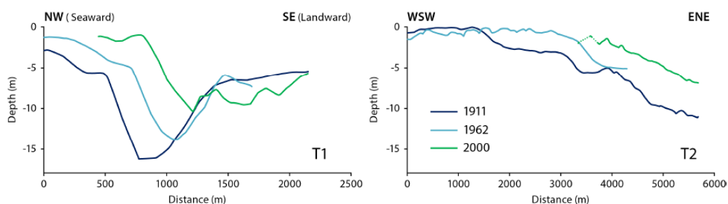
Evolution bathymétrique entre 1911 et 2000 du Banc du Hills perpendiculaire (T1) et parallèle (T2) à la côte (Héquette et al., 2013)
