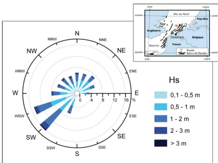
Rose des houles enregistrées à la station de Westhinder au large de 1997 à 2007 (Maspataud, 2011)
