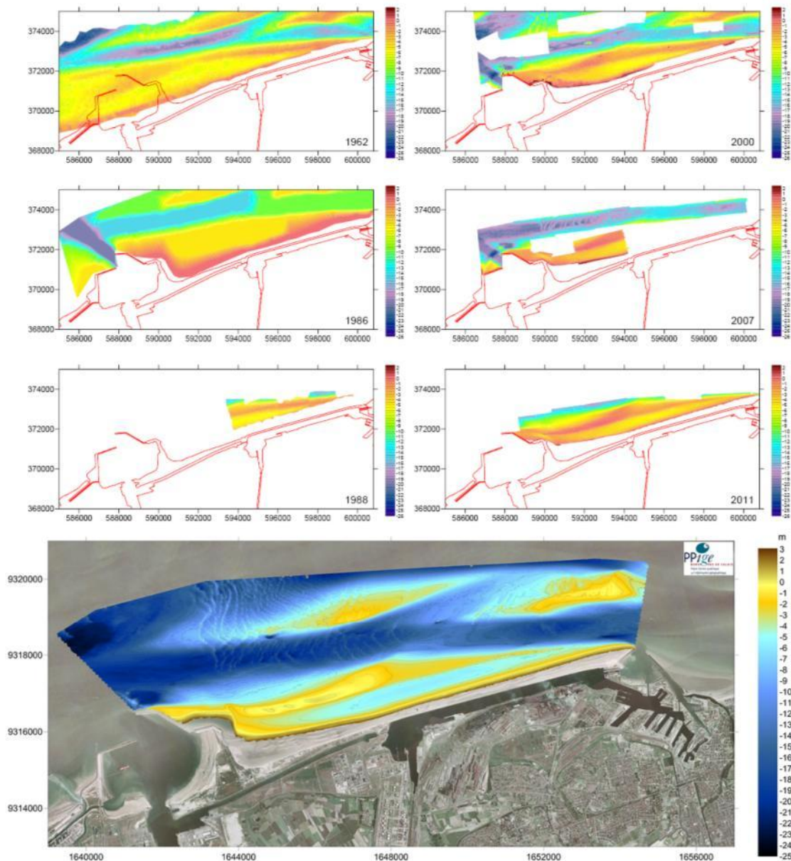
Bathymétries de l'avant-côte de l'UG4 en 1962, 1986, 1988, 200, 2007, 2011 et 2013 (Héquette et al., 2012, 2013 et 2014)
